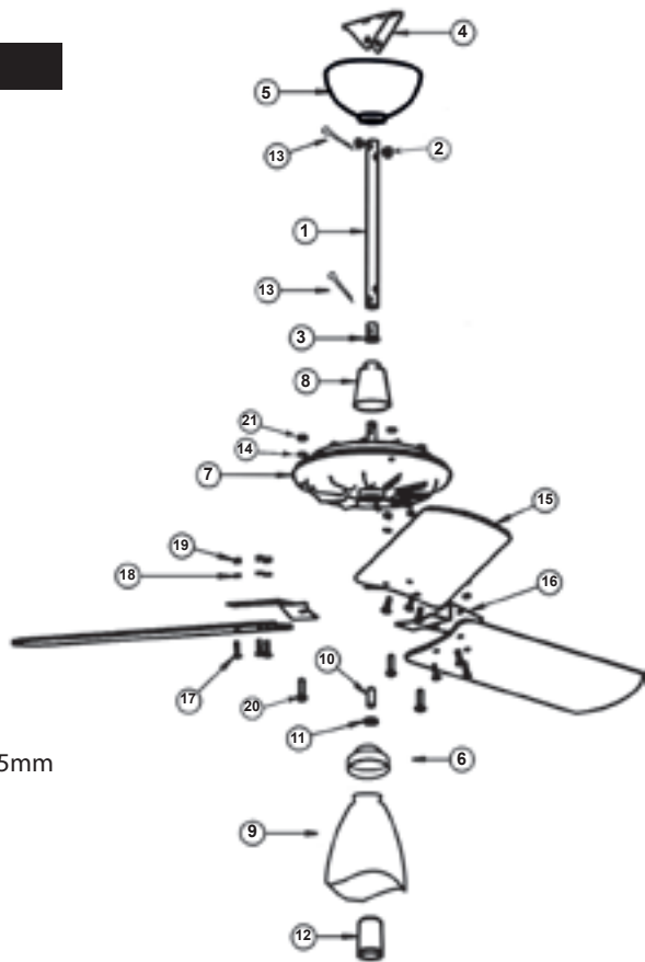
VENTILADOR EXCLUSIVO PARA TETO
